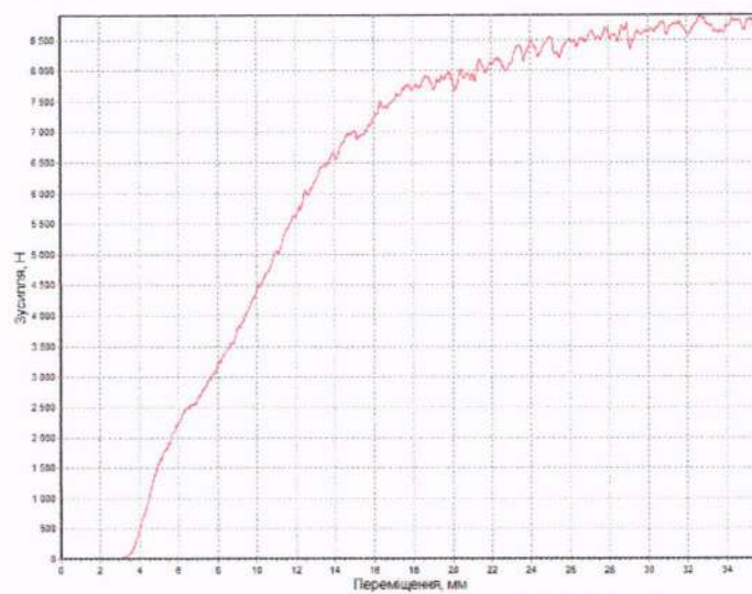
Рисунок 3 – Визначення міцності на стиск виробів теплоізоляційних з піноскла Стандарт ПС
